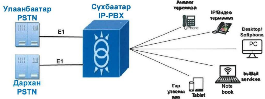
IP-PBX төхөөрөмжийн холболтын схем
