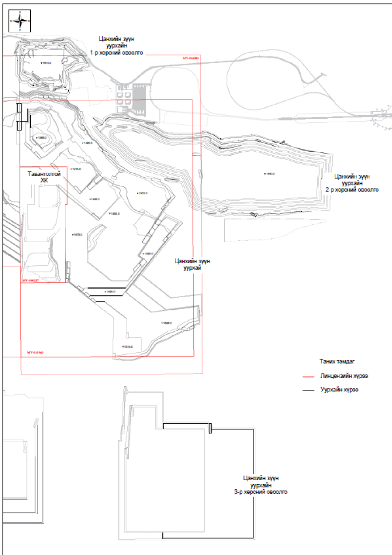
Зураг №1. Уурхайн төлөвлөгөөний зураг
