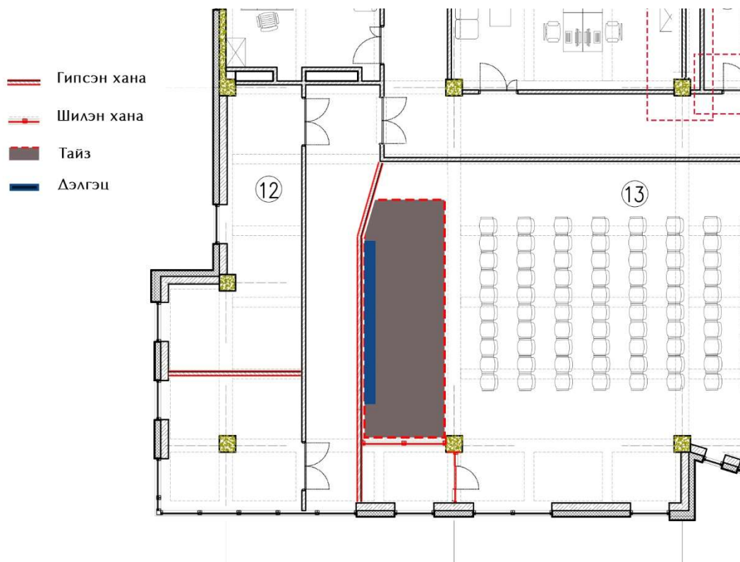
Зураг 1. 5 давхрын барилгын зураг
