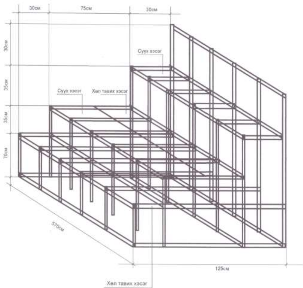
Үзэгчдийн сандалны рамны схем зураг - 1
