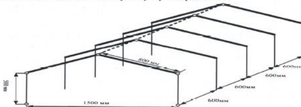
Зураг 01. Туузан дамжуурга дээр суурилагдах тоосруулагчийн схем
