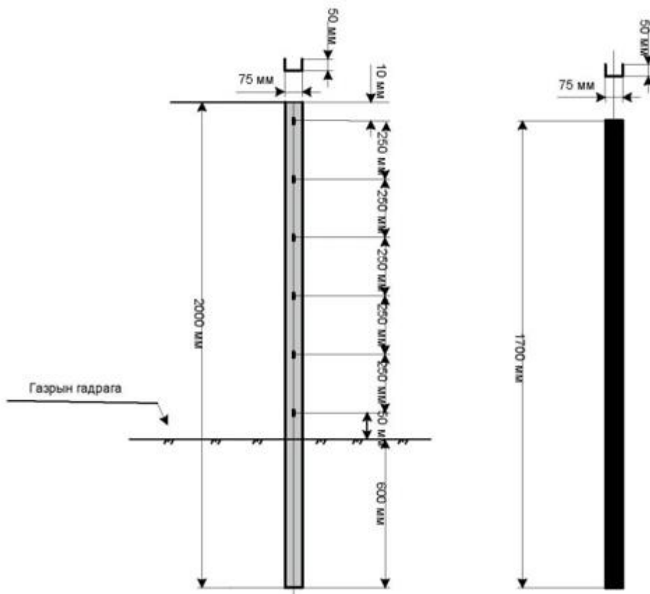
Зураг №1. Хориг хашааны шон болон тулаас шон
