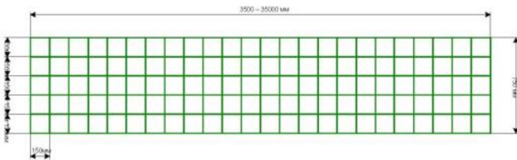
Зураг №2. Хориг хашааны нэмэлт тор
