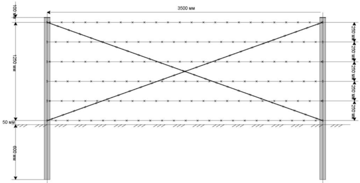
Зураг №4. Өргөст төмөр утсыг татах
