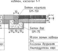
Ногоон байгуулалж, алаг чулуун хавтан, хэсгэлэл 1-1
