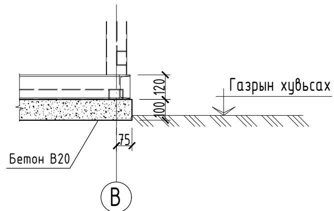
Огтлол 1-1 М1:25
