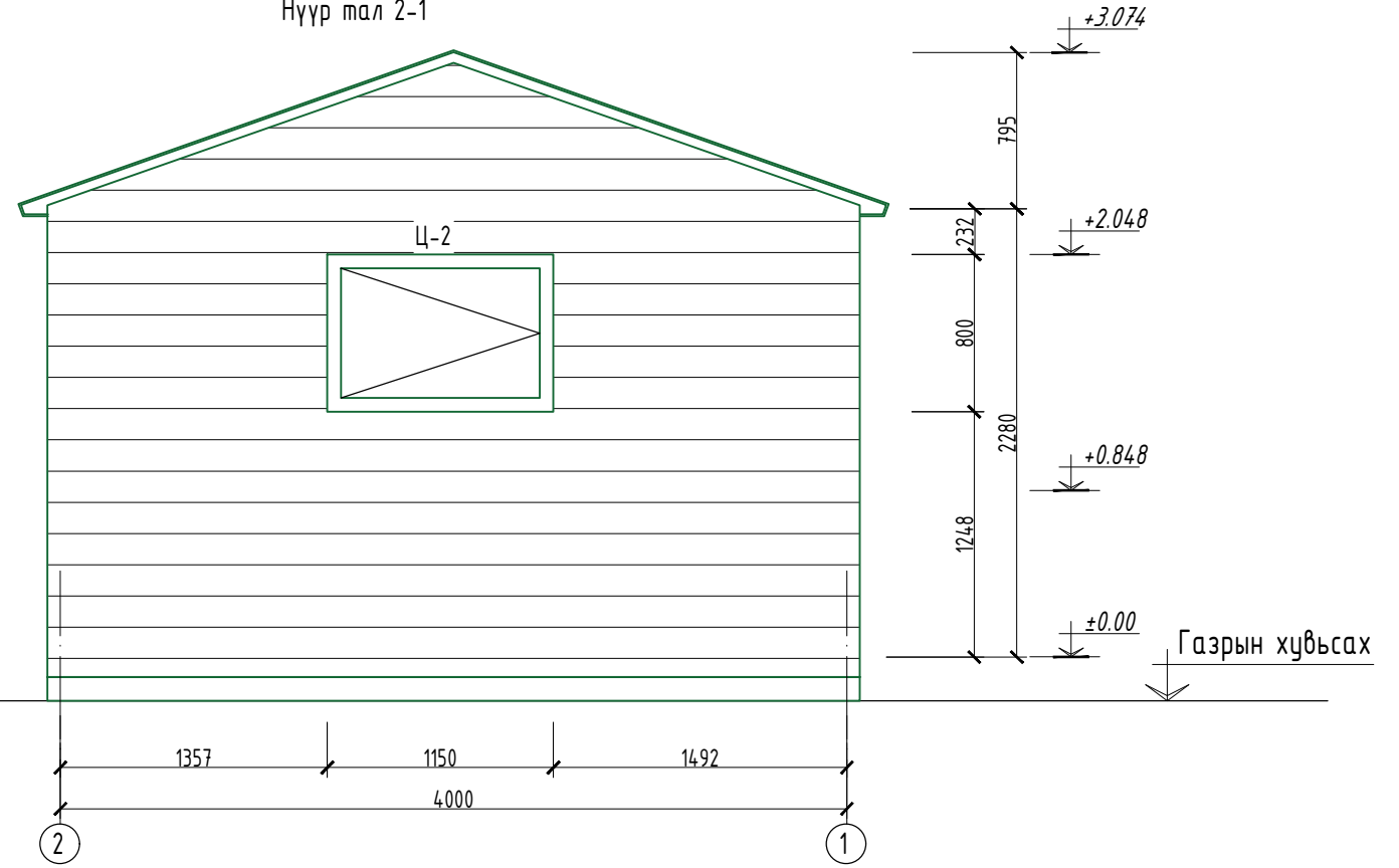
Нүүр тал 2-1
