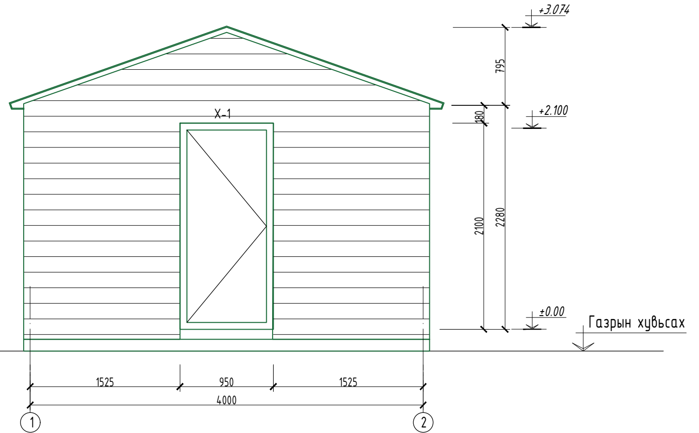
Нүүр тал 1-2
