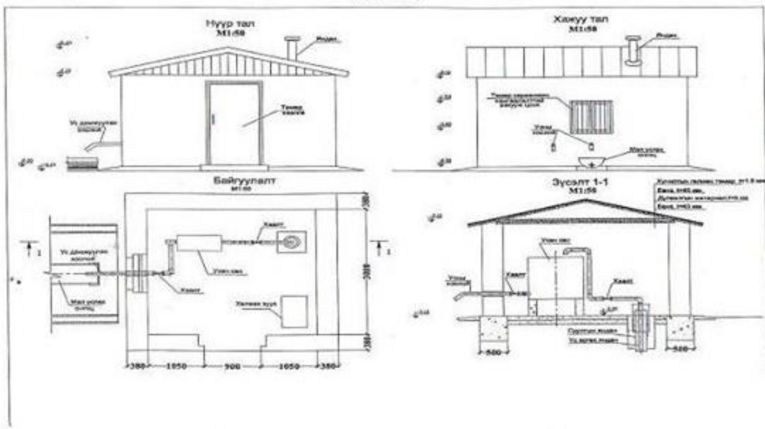
А.1-р зураг – Худгийн барилга
