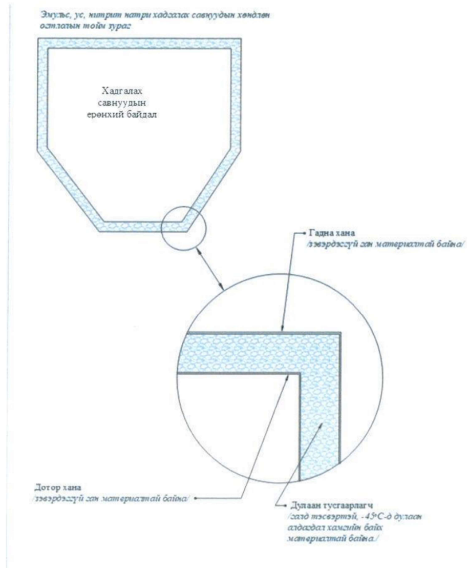
Зураг №3. Эмульс, ус, нитрийн натрийн уусмал хадгалах савны хөндлөн огтлолын тойм зураг
