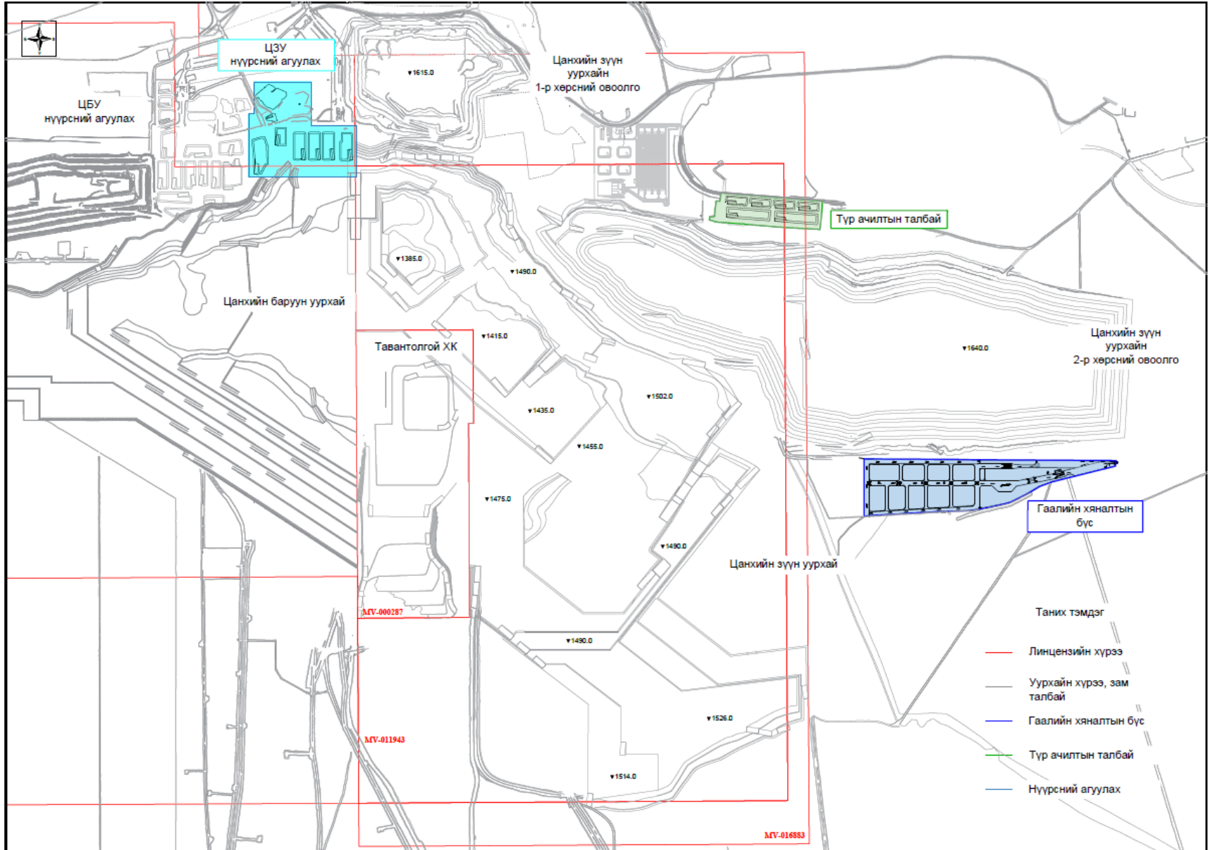
Зураг №1. Нүүрс ачилтын талбайн зураг
