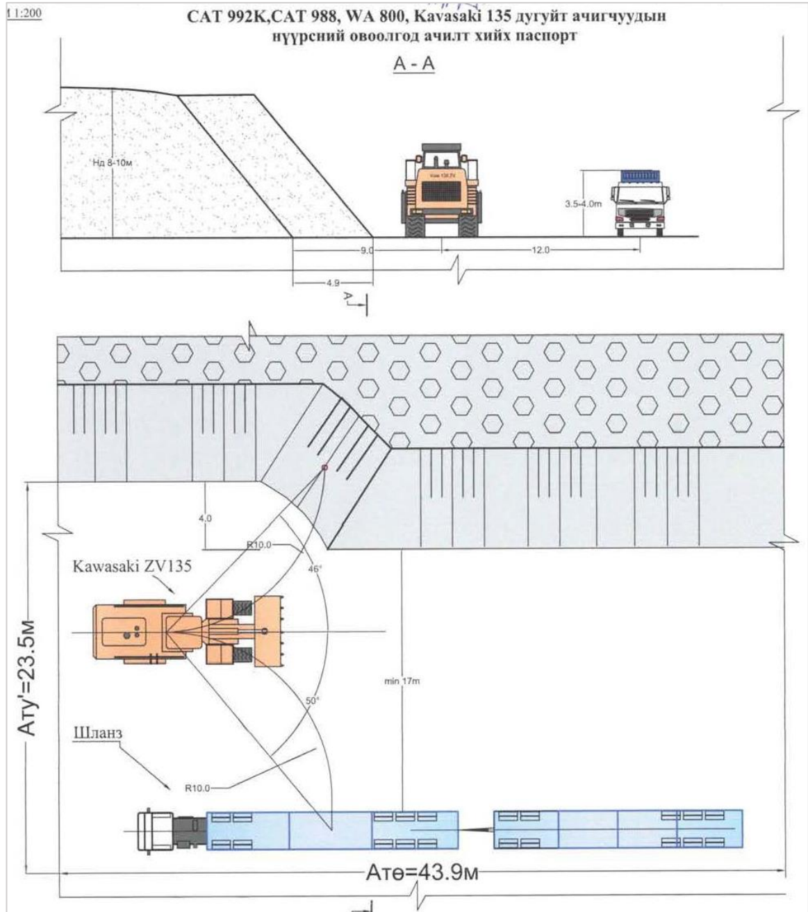
Зураг №2.1. Нүүрсний овоолгод ачилт хийх паспорт
