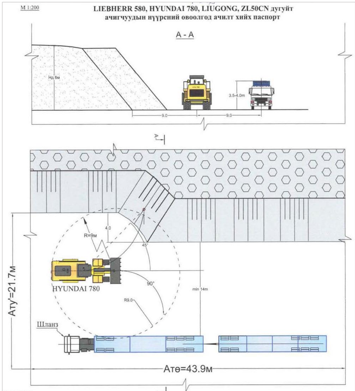
Зураг №2.2. Нүүрсний овоолгод ачилт хийх паспорт
