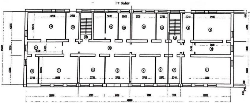
Барилгын дотор план зураг 1-р давхар
