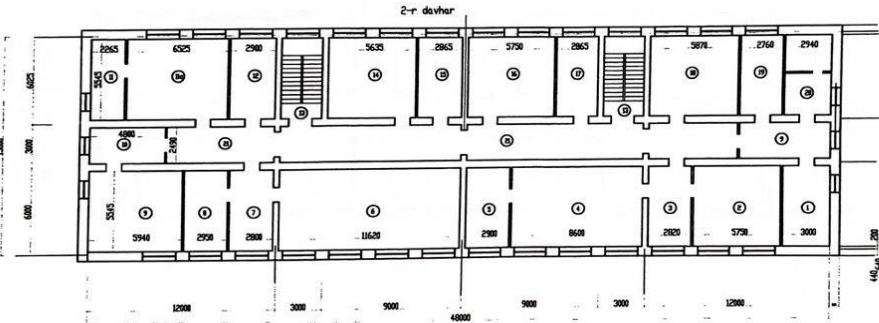
Барилгын дотор план зураг 2-р давхар
