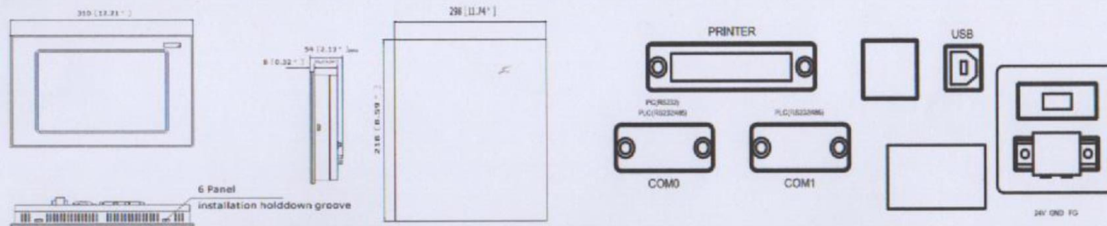
Зураг-1,2,3 /Kinco MT4500T загварын HMI дэлгэцийн хэмжээст зураг, ар талын холболтын портууд/
