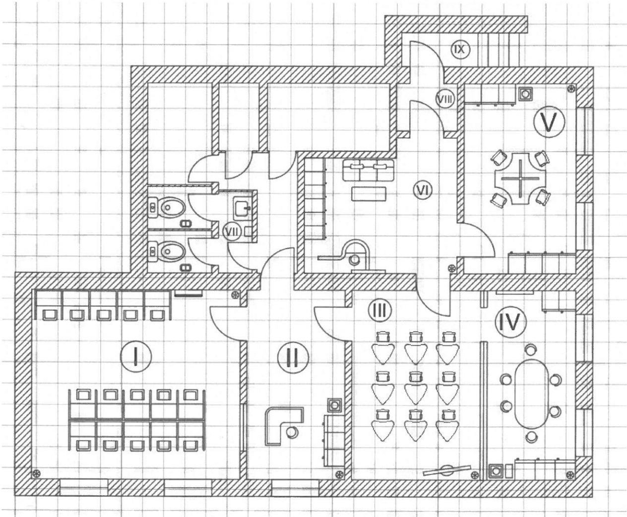
Тавилга тоног төхөөрөмжийн байрлалыг харуулсан план зураг
