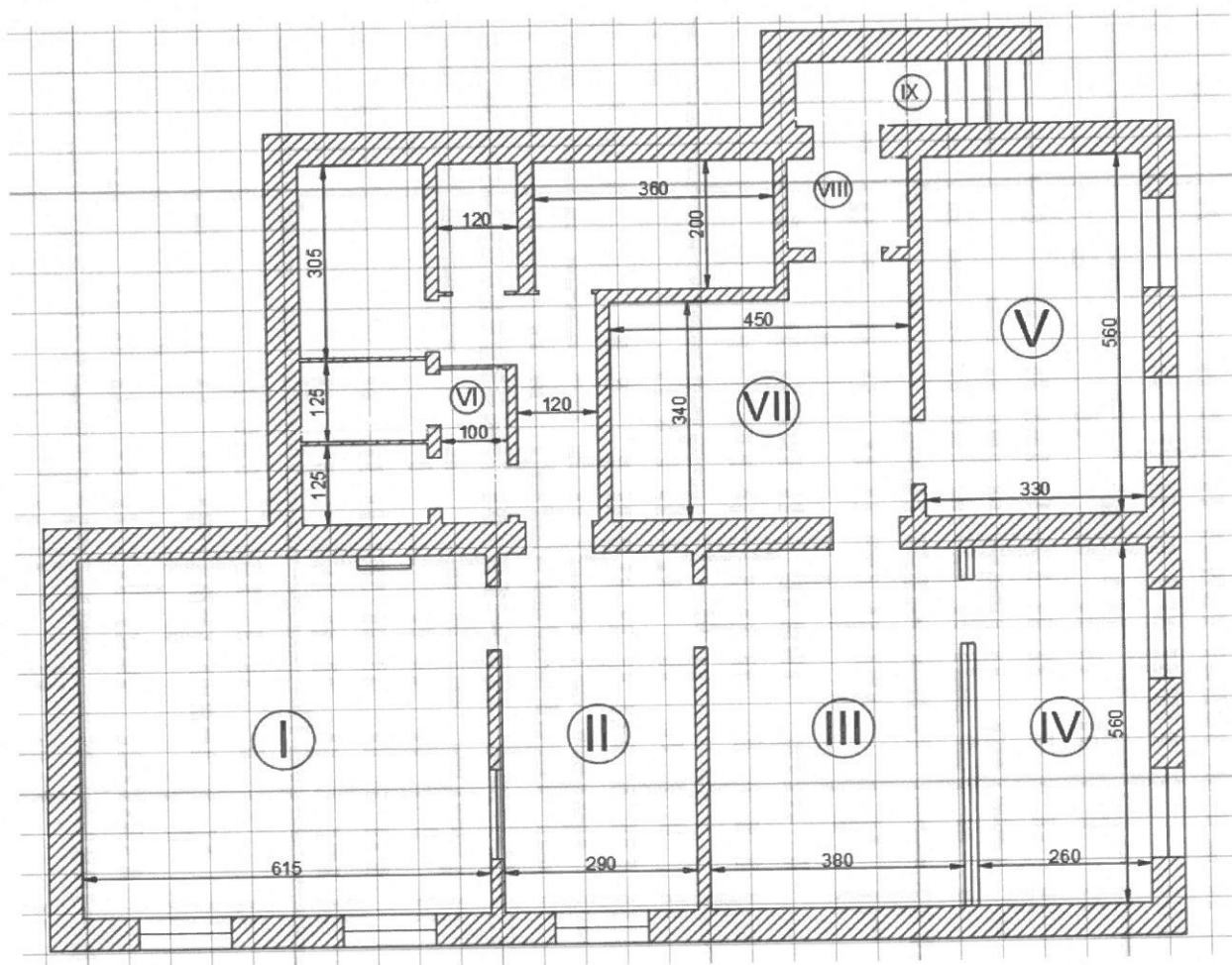
Өрөөнүүдийн хэмжээ заасан план зураг
