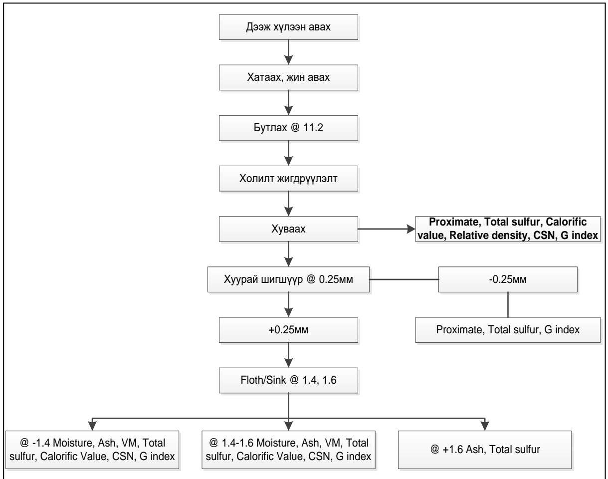
Зураг-1. Баяжуулалтын анхан шатны туршилт шинжилгээний схем, шинжилгээний төрөл
