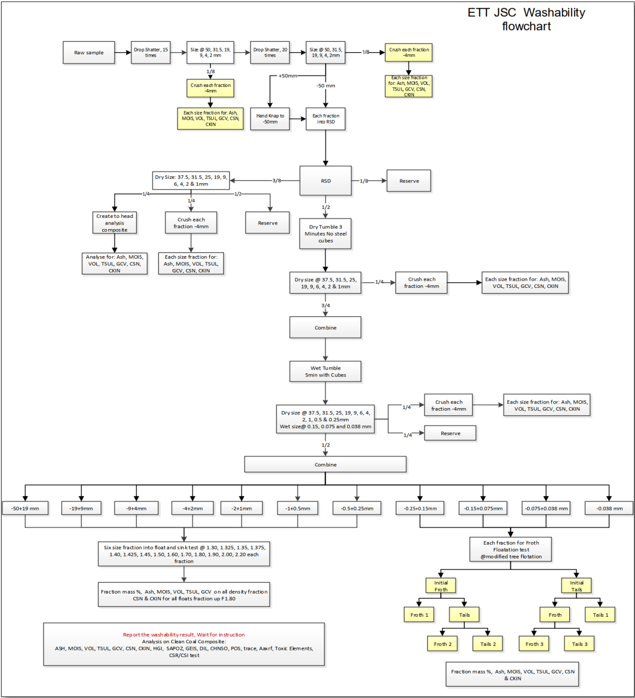
Зураг-2. Гүн баяжуулалтын туршилт шинжилгээний схем, шинжилгээний төрөл
