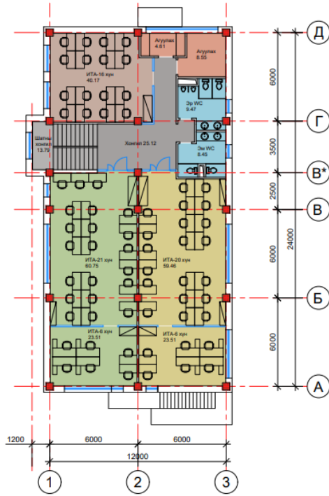
2 ДУГААР ДАВХРЫН БАЙГУУЛАЛТ M1:150
