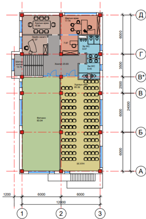
4 ДҮГЭЭР ДАВХРЫН БАЙГУУЛАЛТ M1:150
