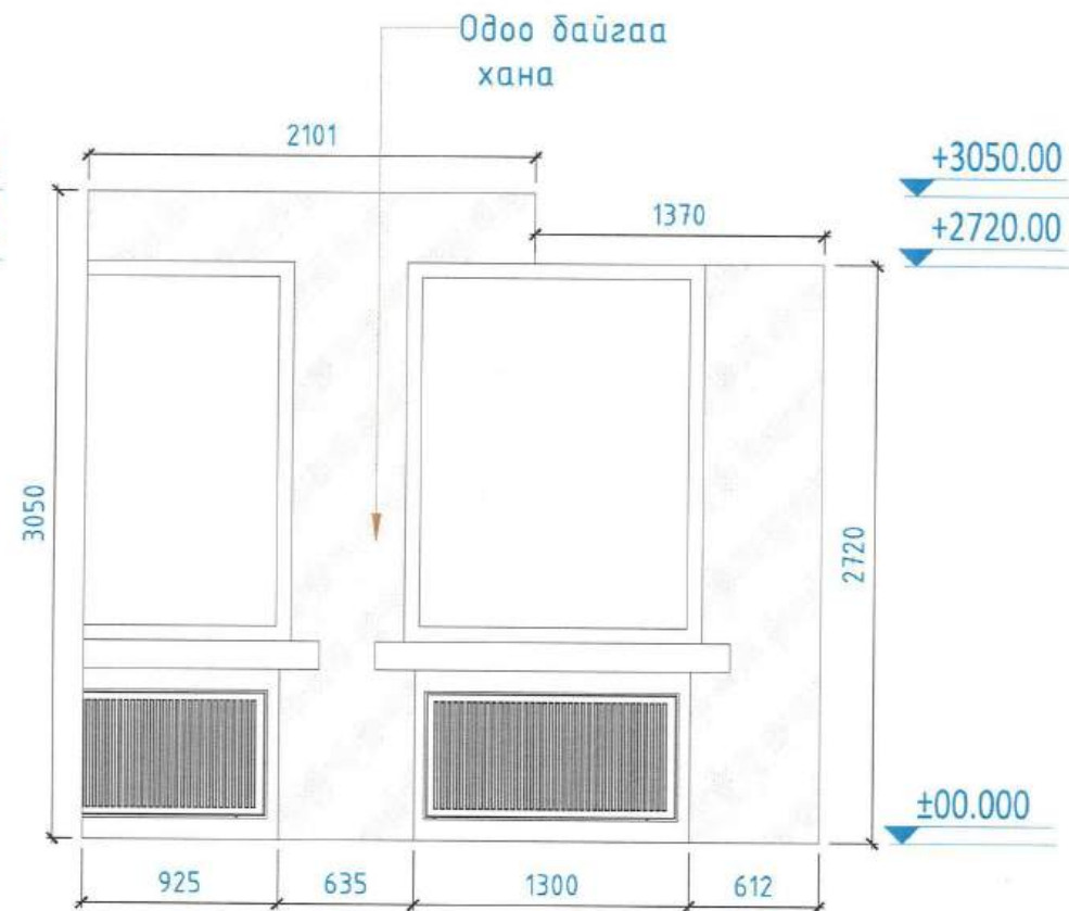
ХАНЫН ДЭЛГЭЭС-19 M 1:50 IN A3 FORMAT
