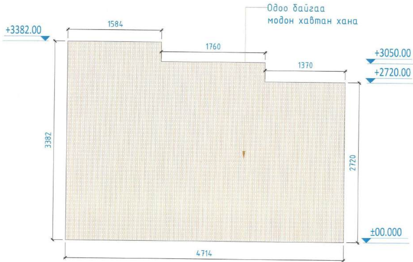
ХАНЫН ДЭЛГЭЭС-18 M 1:50 IN A3 FORMAT
