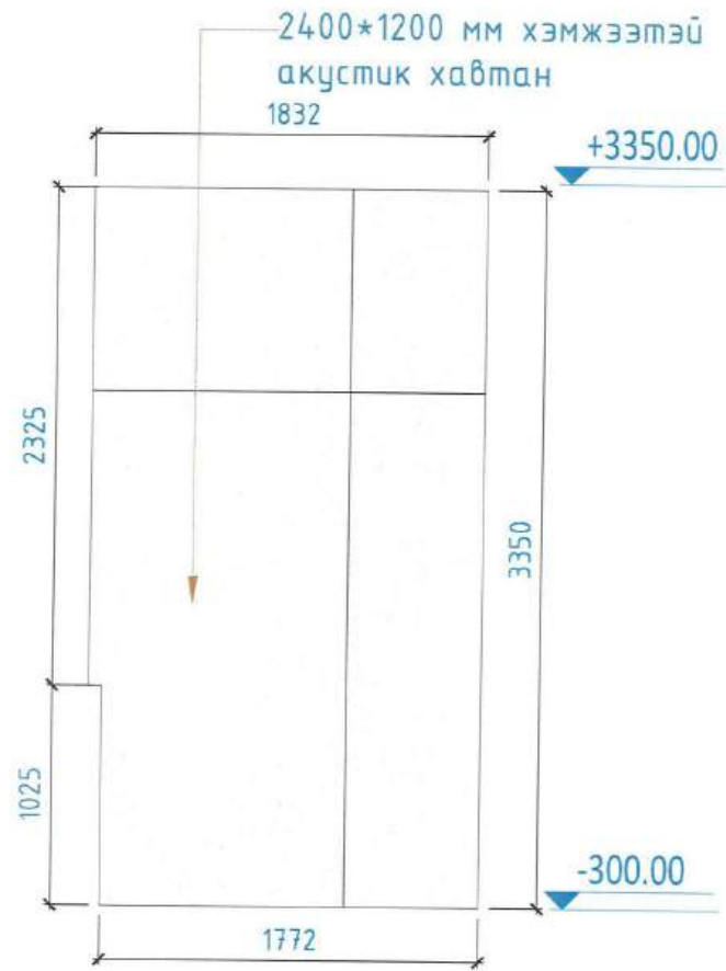
ХАНЫН ДЭЛГЭЭС-8 M 1:50 IN A3 FORMAT
