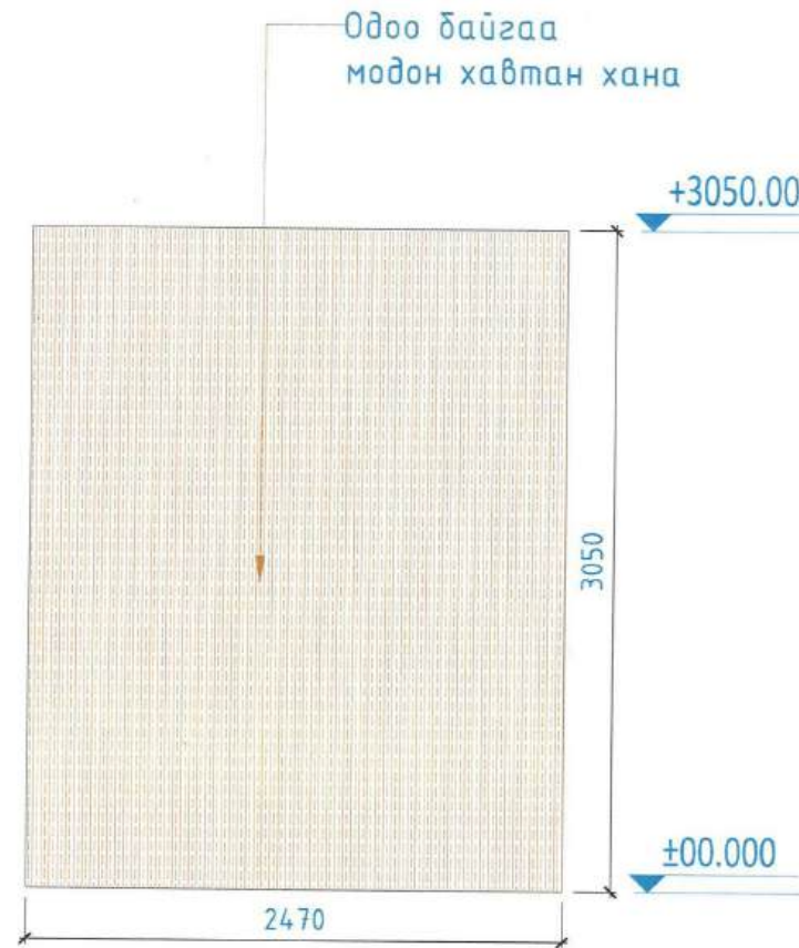
ХАНЫН ДЭЛГЭЭС-2 M 1:50 IN A3 FORMAT
