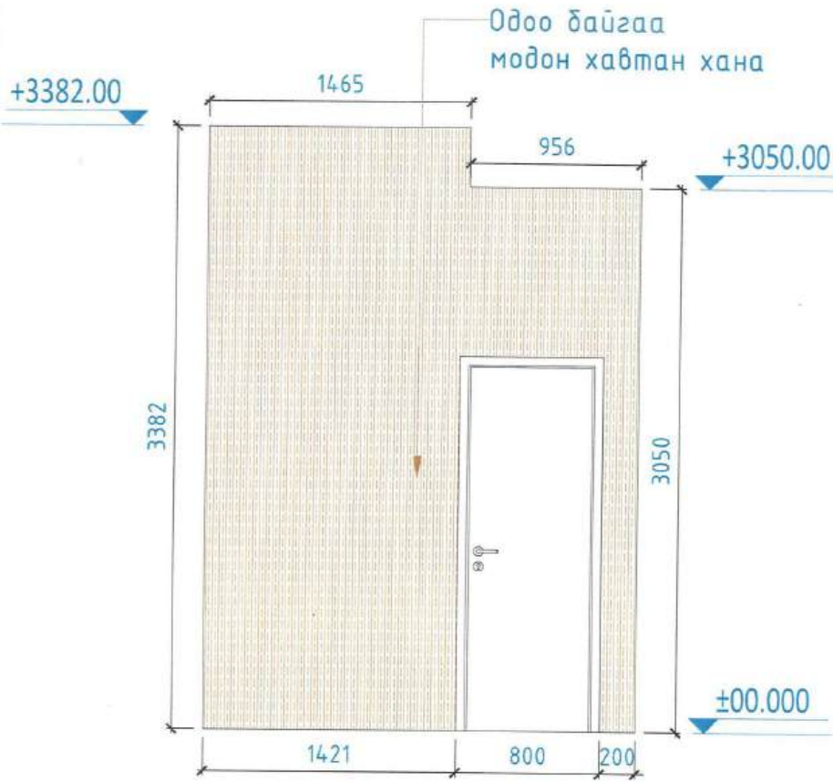
ХАНЫН ДЭЛГЭЭС-4 M 1:50 IN A3 FORMAT
