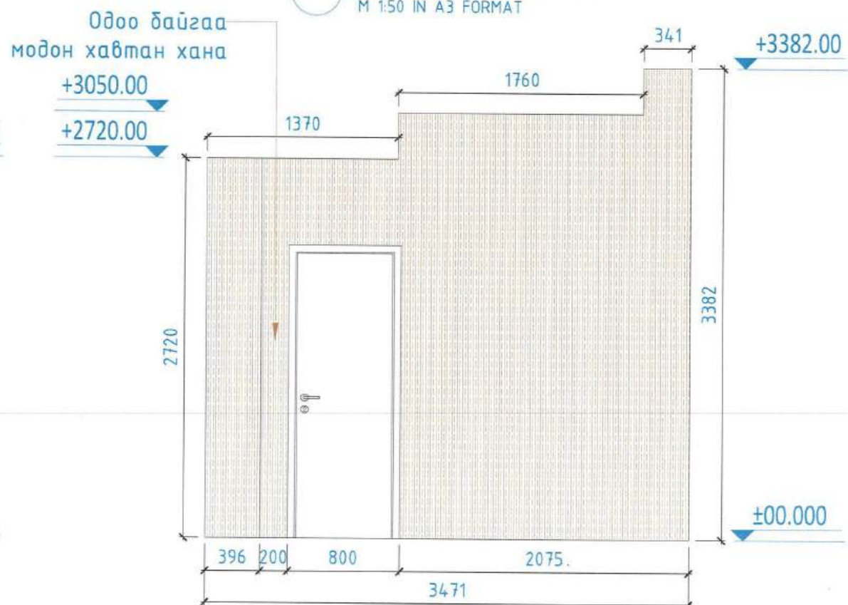
ХАНЫН ДЭЛГЭЭС-19 M 1:50 IN A3 FORMAT
