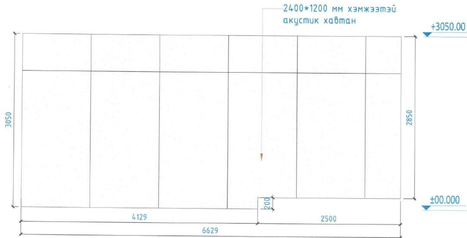
ХАНЫН ДЭЛГЭЭС-12 M 1:50 IN A3 FORMAT
