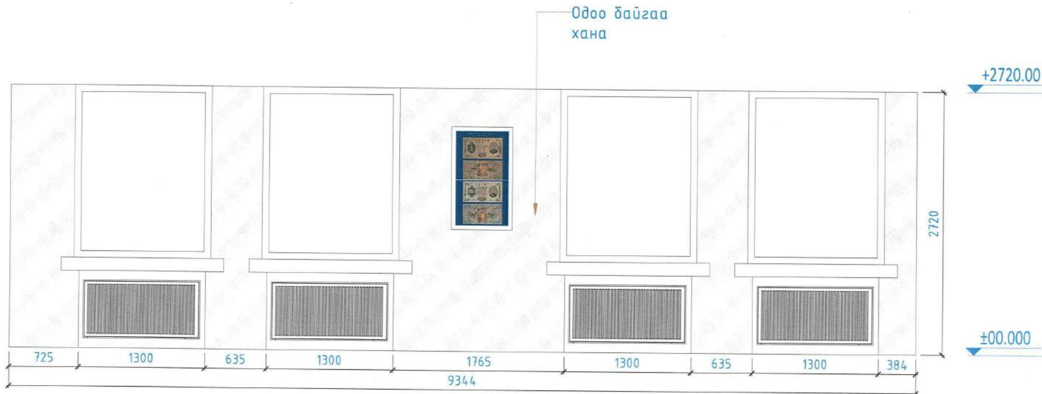
ХАНЫН ДЭЛГЭЭС-4 M 1:50 IN A3 FORMAT
