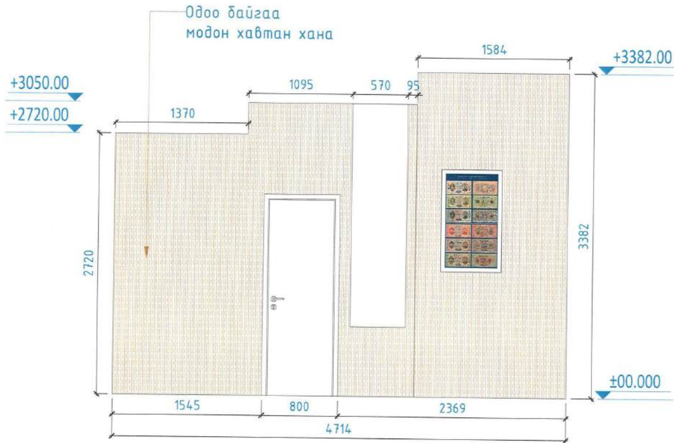
ХАНЫН ДЭЛГЭЭС-6 M 1:50 IN A3 FORMAT
