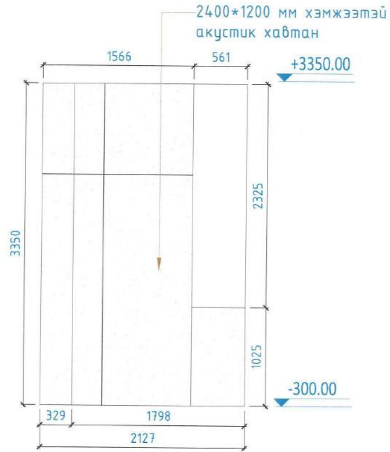
ХАНЫН ДЭЛГЭЭС-7 M 1:50 IN A3 FORMAT
