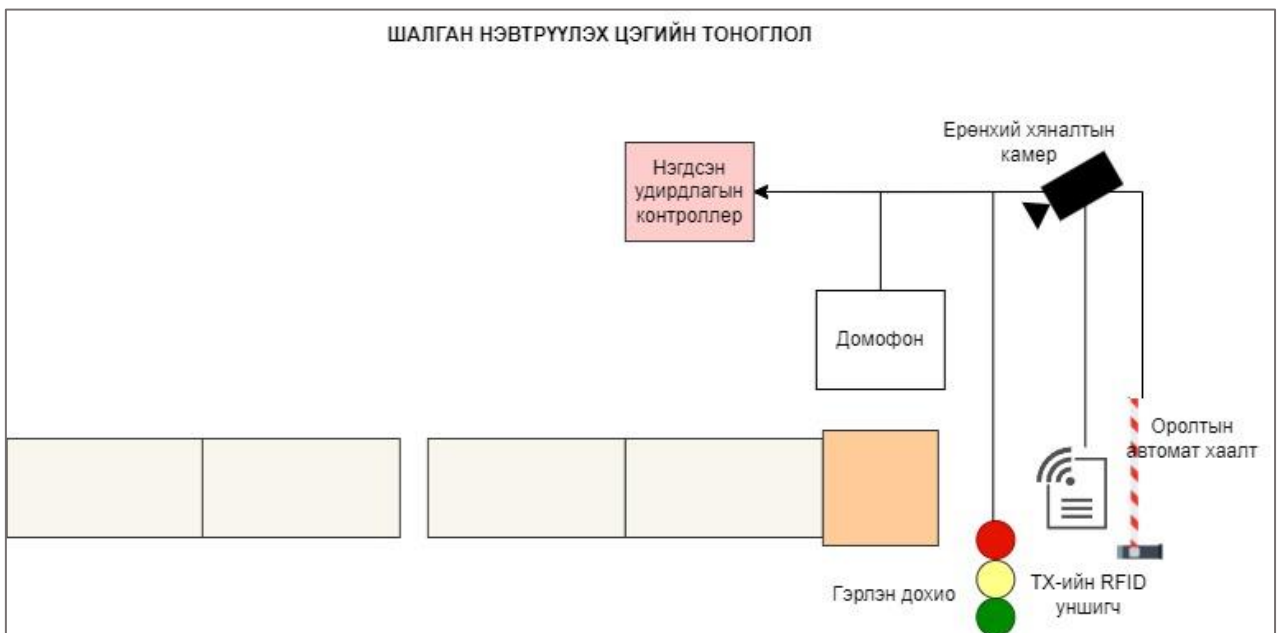
Зураг 5. Гаалийн хяналтын бүсийн оролт, гаралтын нэвтрэх цэгийн тоноглол
