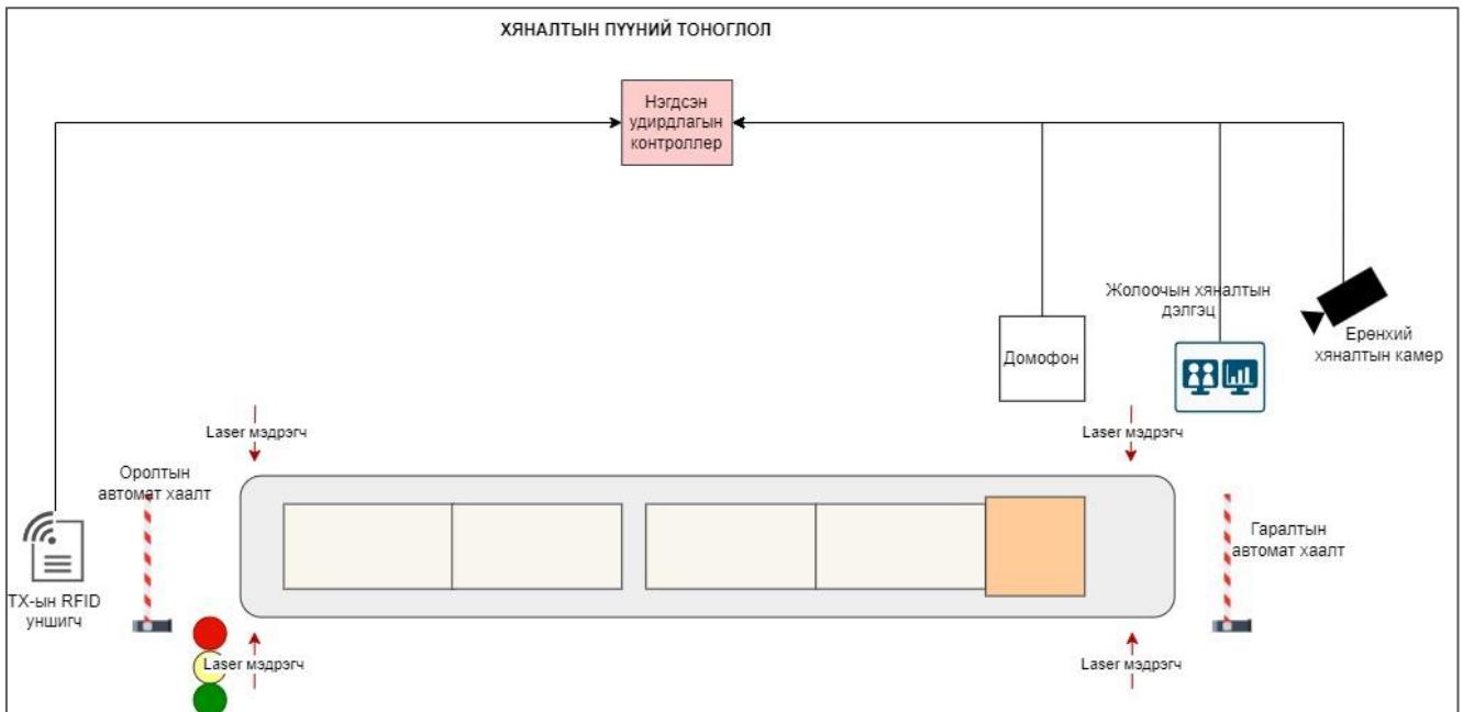
Зураг 4. Хяналтын авто жингийн тоноглол
