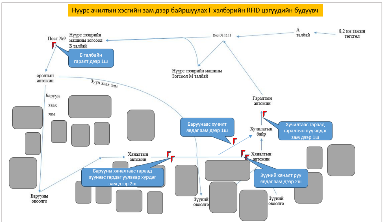
Зураг 6. НАХ хэсэгт RFID уншигч байрлуулах цэгүүд
