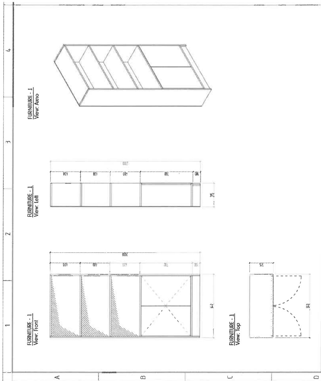
Зураг 9. Номын тавиурны нарийвчилсан хэмжээ
