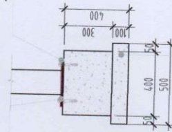
Анкер доолт
