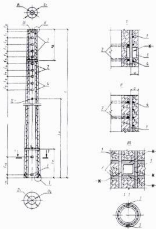
Төмөрбетон конусан шонгийн бэхэлгээний хийцийн хэмжээс, мм
