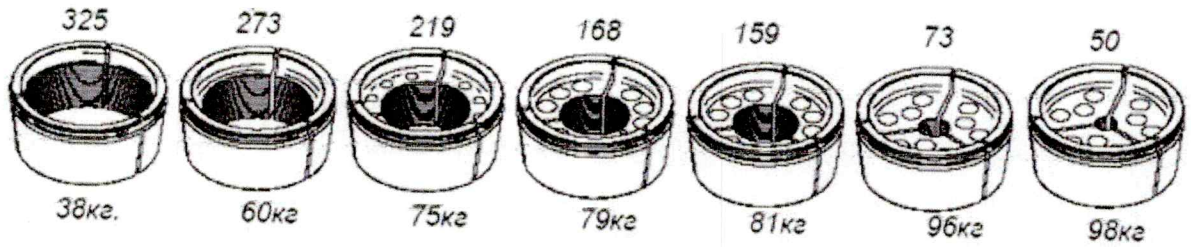
Яндан хоолой сугалах плашка Зураг №3
