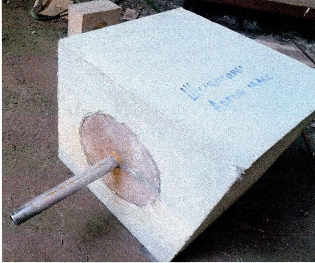
АРГОНЫ МАССЫН ЗУРАГ ASSEMBLED PURGING PLUG, SEATING BLOCK'S PICTURE
