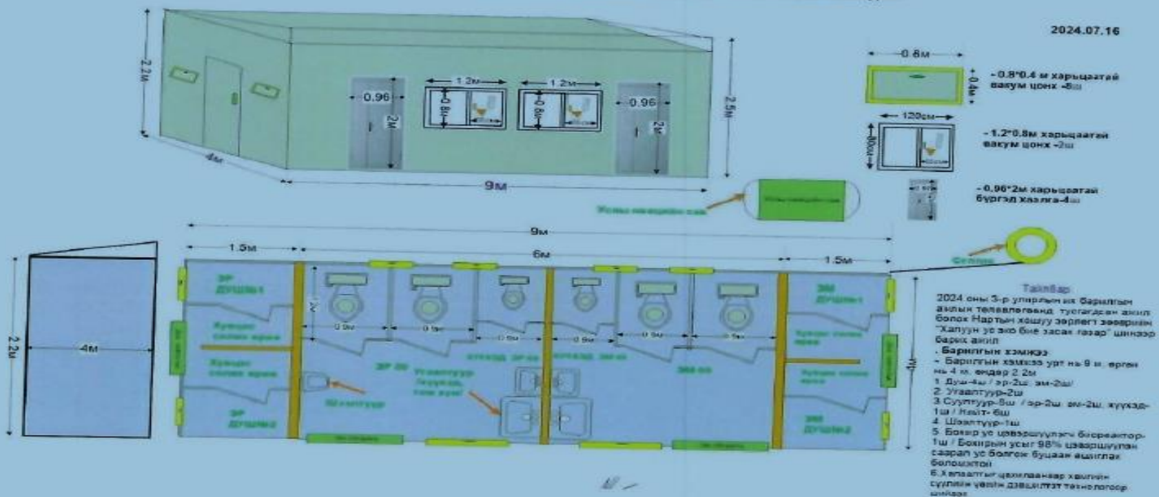
УБТЗ-ын Замын 4-р ангийн Нартын хошуу зөрлөгт зөөврийн "Халуун ус, Эко 00" барих схем зураг:
