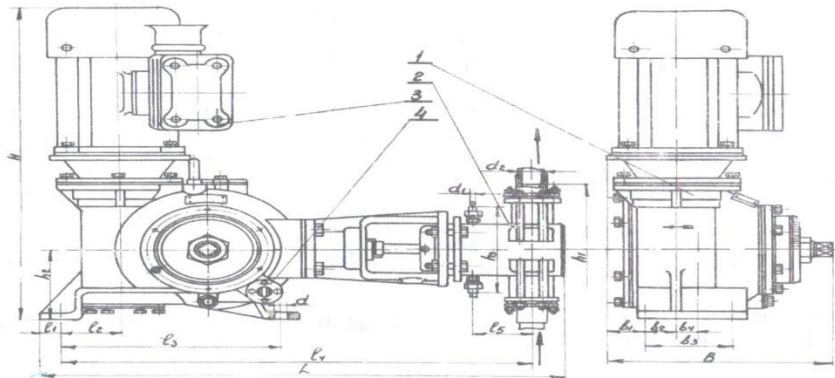
НД-- насосны ерөнхий байдал 1-редуктор , 2-гидравлик хэсэг 3 - цахилгаан хөдөлгүүр
